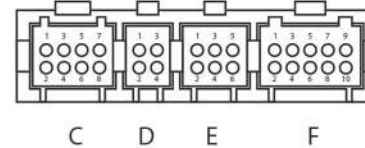
Схема разъемов подключения.
