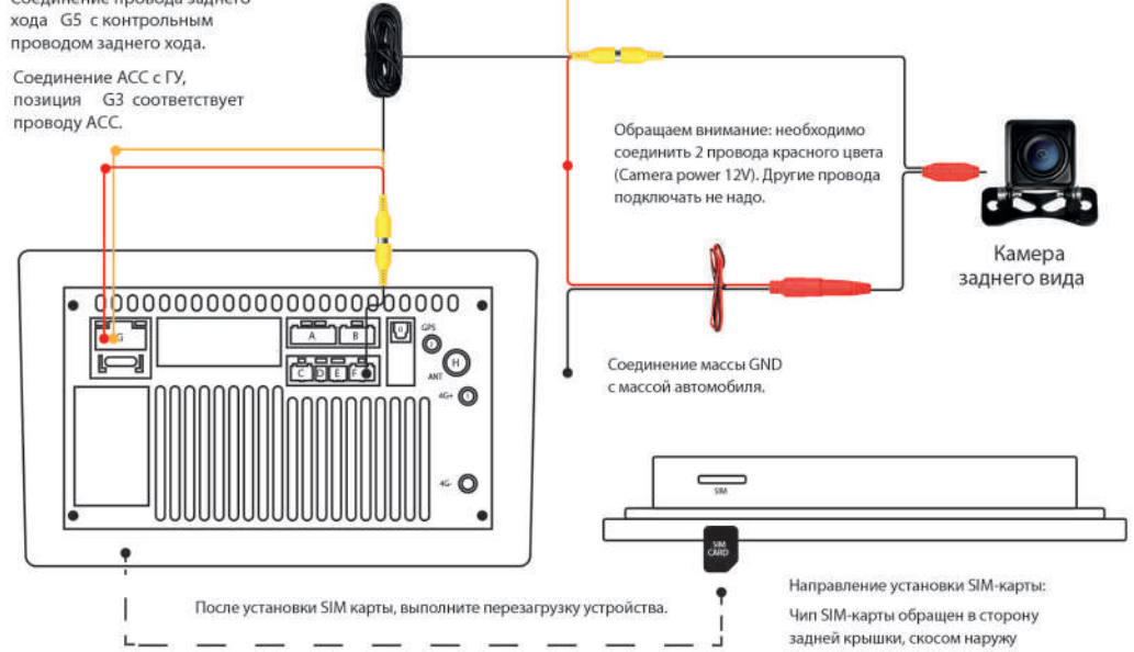
Схема разъемов подключения.
