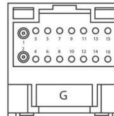
Кабель основного питания.
