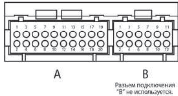
Схема разъемов подключения.
